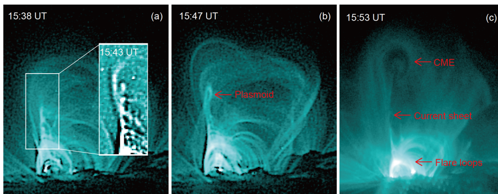
图2 (网络版彩色)SDO卫星AIA 131 Å波段(Fe XXI发射线,形成温度约10 MK)于2013年5月13日观测到的日冕物质抛射 [84] 。(a)爆发前的电流片结构,小图通过增强精细结构显示电流片撕裂为多个等离子体团;(b)爆发初始时刻,电流片顶端存在一个较大的等离子体团;(c)爆发结构在内日冕呈现椭圆形,身后拖出一条电流片与耀斑环相连
