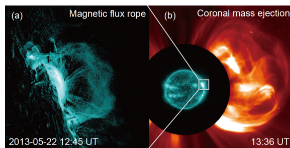
图3 (网络版彩色)磁绳的爆发.(a) SDO卫星AIA 131 Å波段观测到的处于爆发过程中的高温磁绳结构;(b) 131 Å成像与SOHO卫星LASCO-C2白光日冕的合成图,显示磁绳爆发导致的CME [91]
